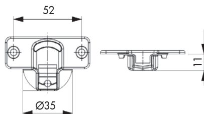
Kućište baglame - ugradnja vijcima
